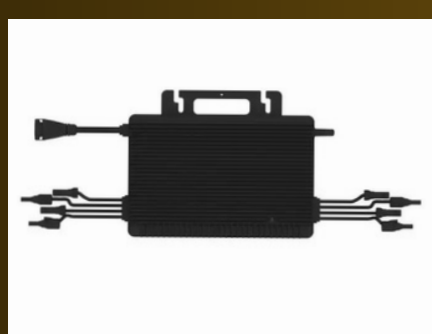
Micro Inverter Hoymiles HMT-2000-4T จำนวน 2 เครื่อง
